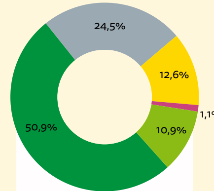
Verbleibender Energieträgermix
